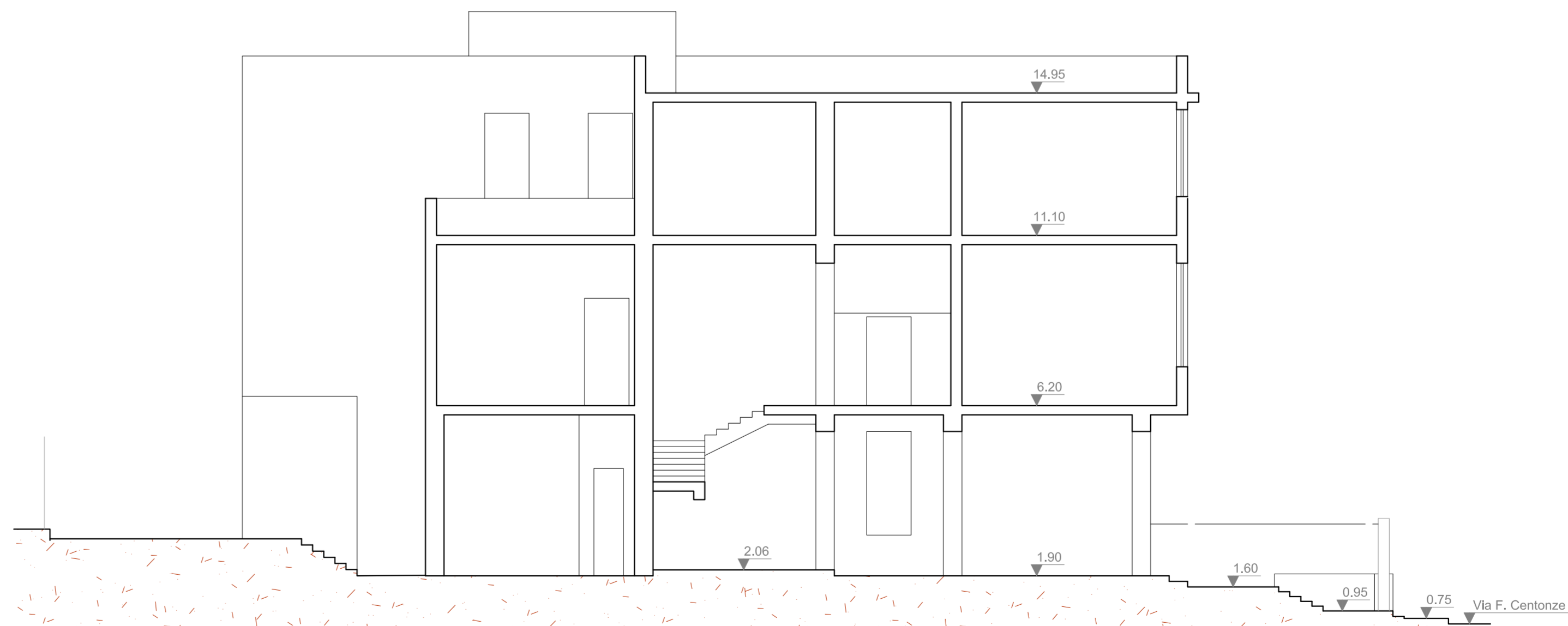
Sezione B-B
