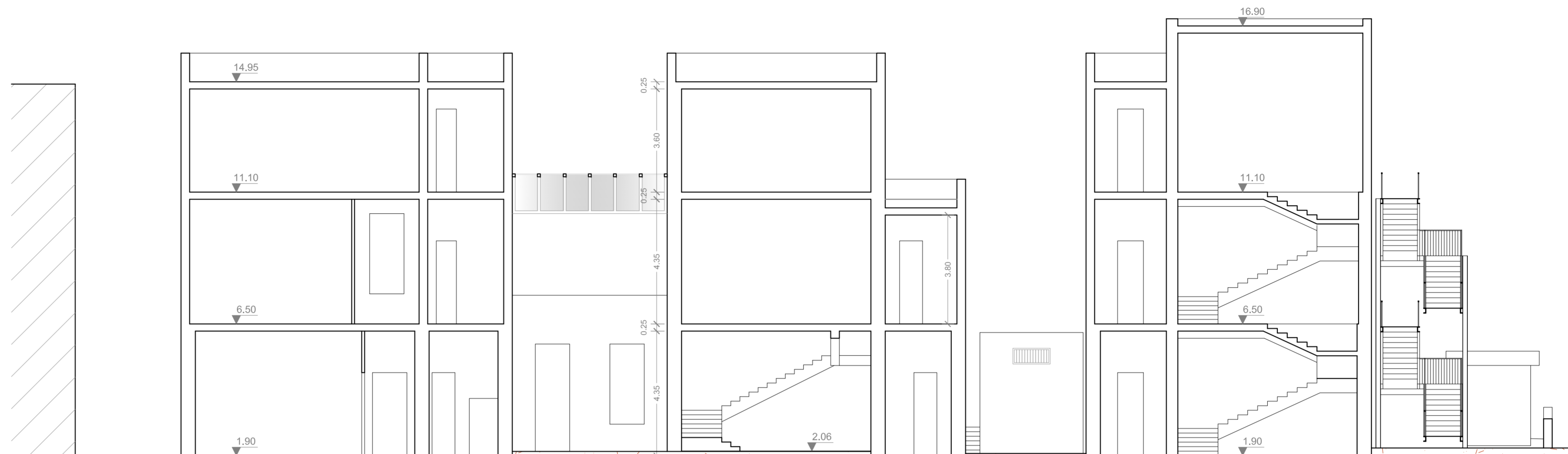
Sezione A-A
